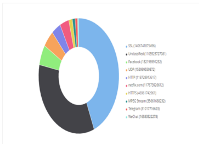
Primeras 10 aplicaciones
