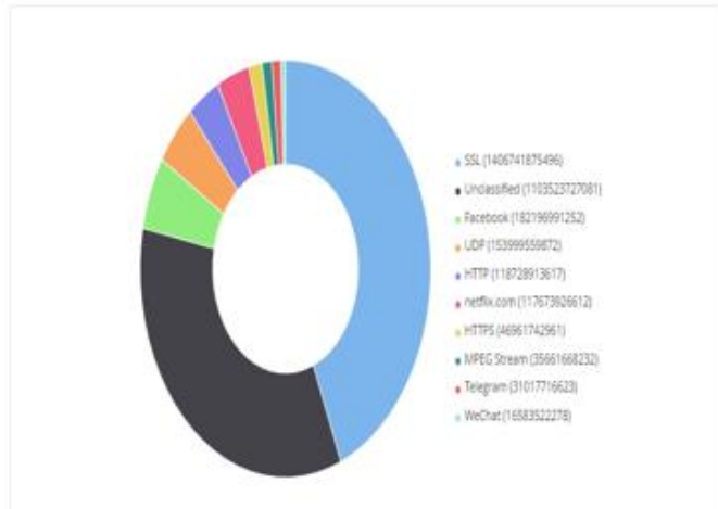
Primeras 10 aplicaciones
